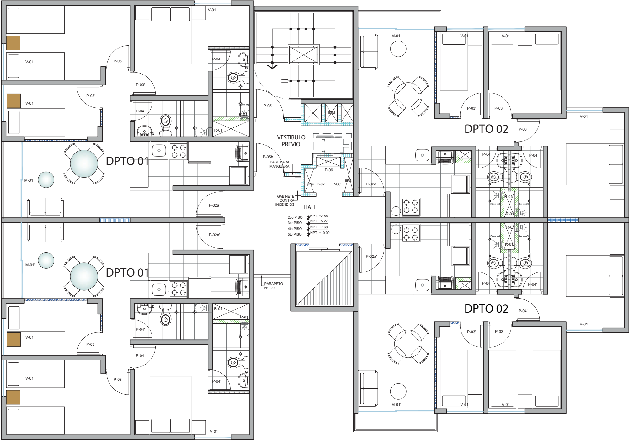
PLANTA TIPICA DEL 02 AL 06 PISO - TORRE 01 AL 04
