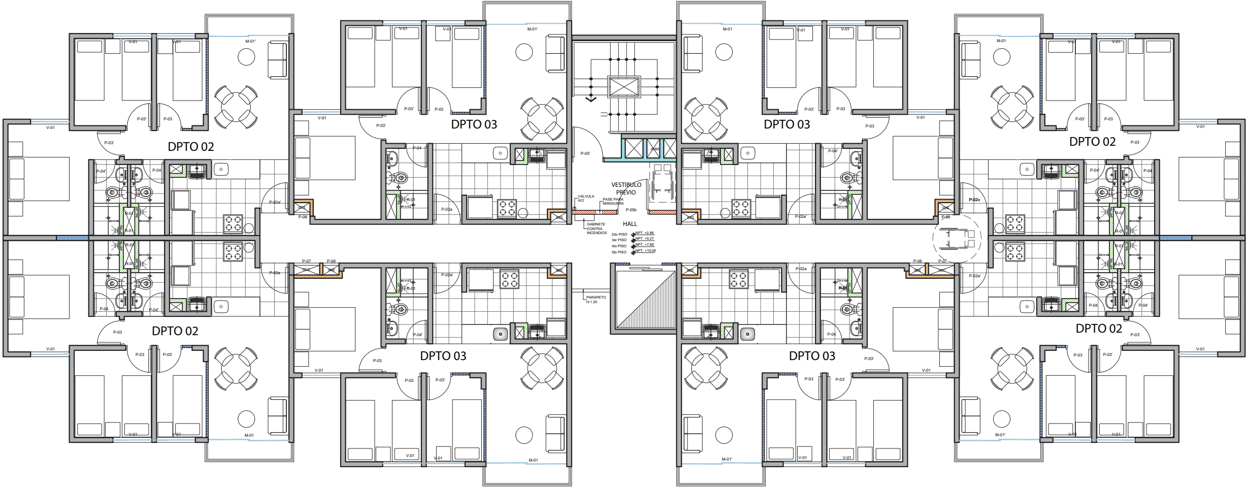
PLANTA TIPICA DEL 02 AL 06 PISO - TORRE 05
